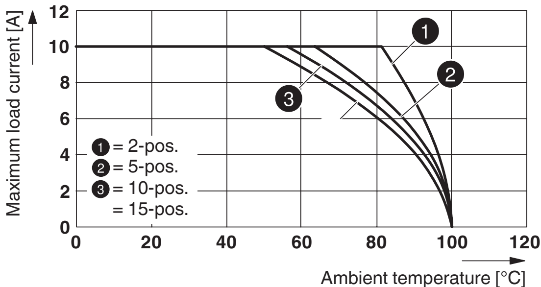
Courbe de derating pour ST 2,5-4L/1P, ST 2,5-4L/2P et pour toutes les variantes de connecteurs SP...
