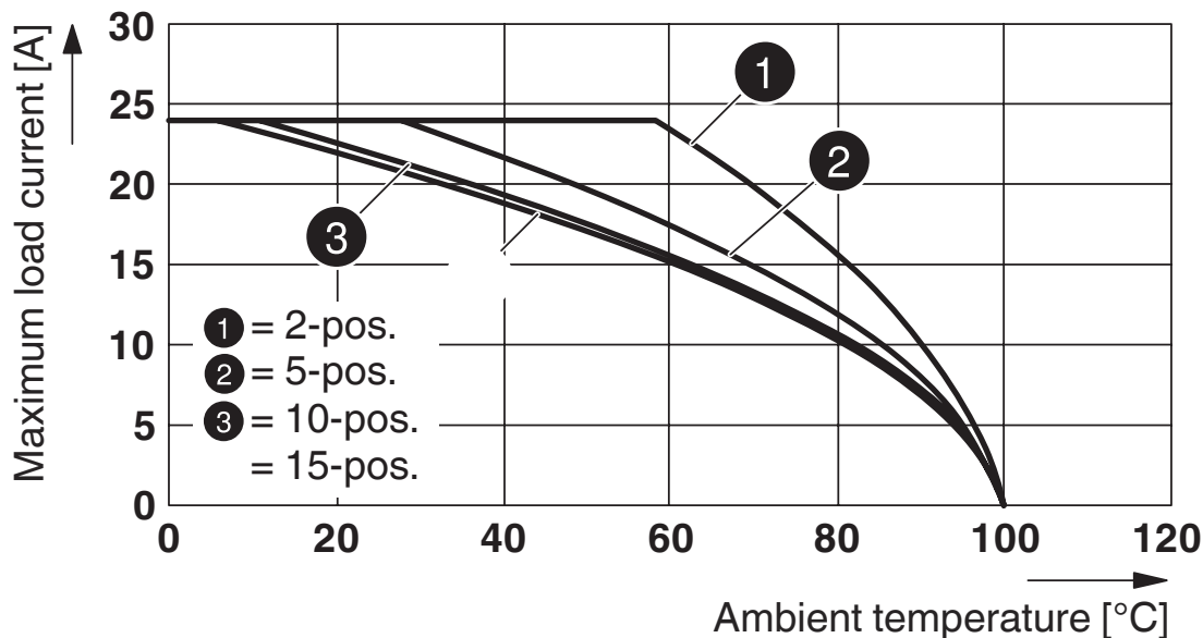
Courbe de derating pour ST 2,5-QUATTRO/2P, ST 2,5-QUATTRO/4P et pour toutes les variantes de connecteurs SP...
