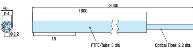
E32-ET11R
