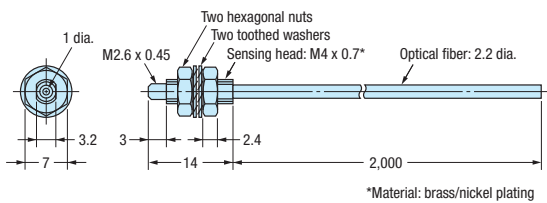
E32-ET11R
