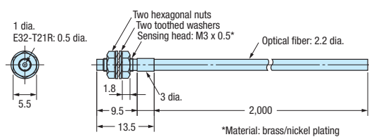
E32-ET51
