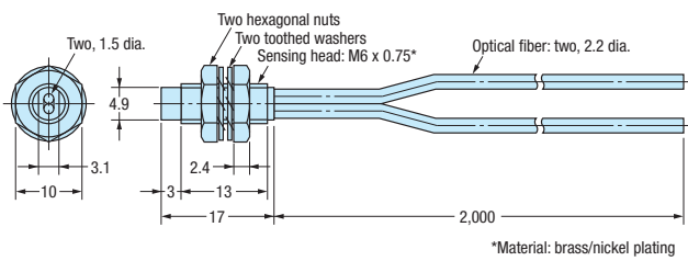
E32-EDS24R
