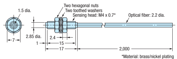
E32-ETC220 2M
