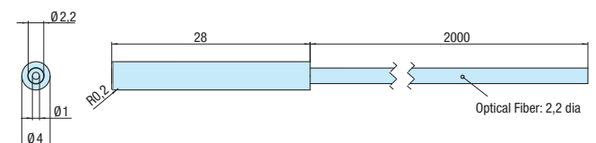
E32-ETC220 2M
