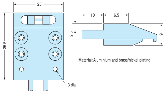
E32-ET11F
